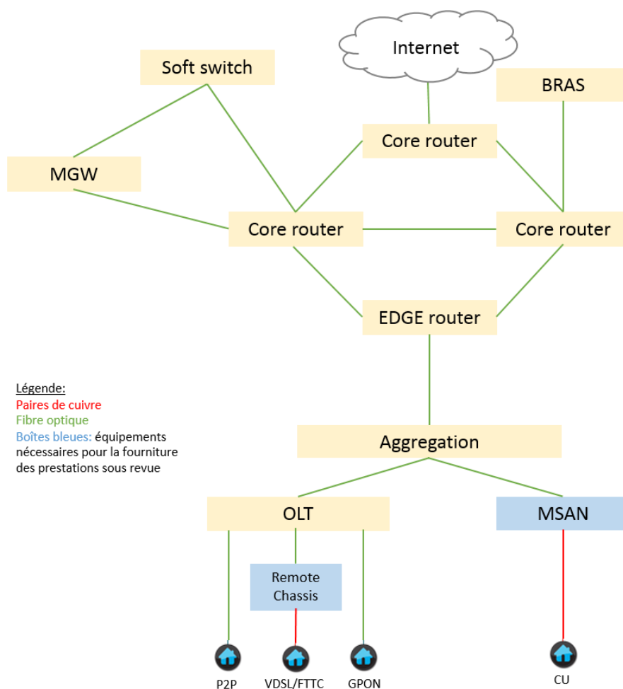
Graphique 6-2 Hiérarchie des catégories d'éléments de réseau [source: ILR, « Model methodology », avril 2014]
