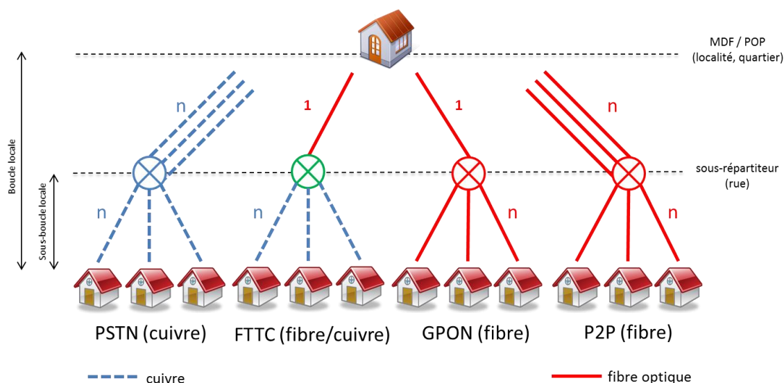
Graphique 6-4 Les types d'infrastructure du réseau d'accès [Source : ILR]
