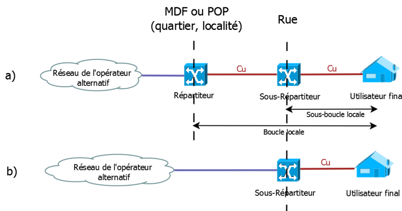
Graphique 2-1: Illustration des prestations de dégroupage de la boucle et de la sous-boucle locale de la paire de cuivre [Source: ILR]
