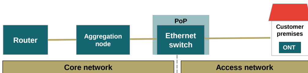
Figure 21. FTTH - P2P
