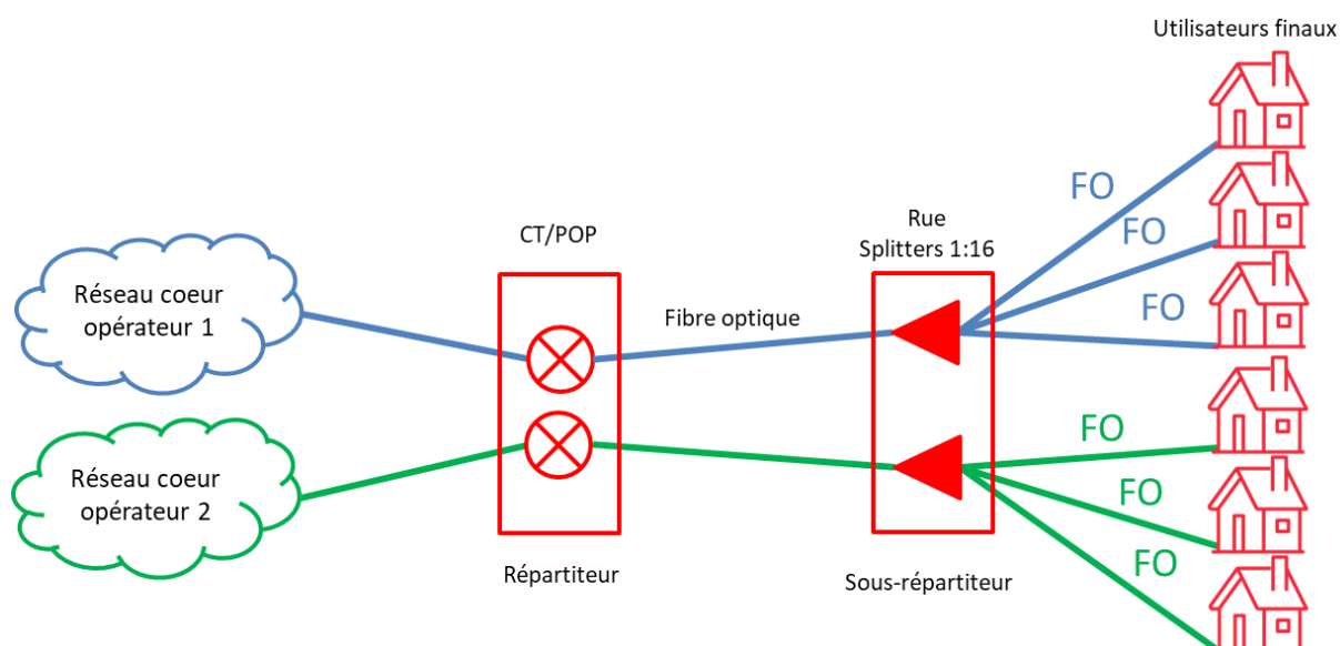
Graphique 4-1 : Dégroupage de la fibre optique dans un scénario FTTH-P2MP (Source : ILR, 2024)
