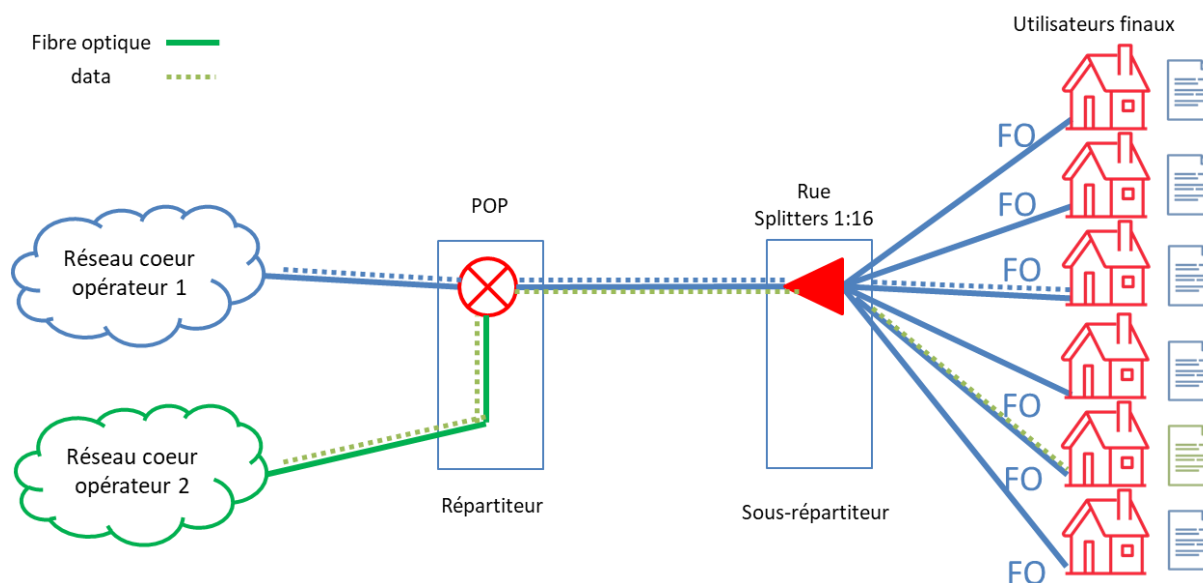
Graphique 4-2 : Schéma de principe VULA (Source : ILR, 2024)
