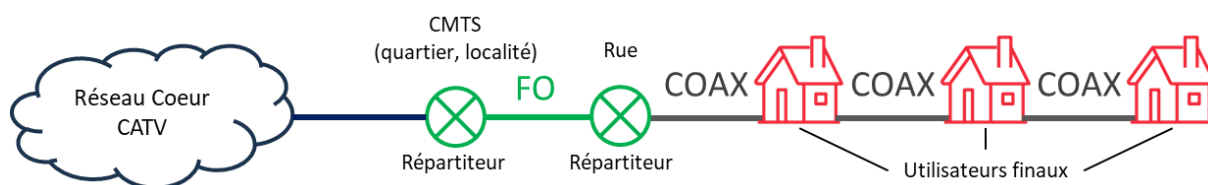
Graphique 2-10 : Configuration d'un réseau FTTLA
