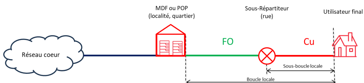
Graphique 2-2 : Représentation graphique d'un réseau partiellement en cuivre
