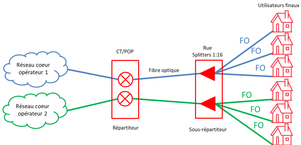
Graphique 4-8 : Schéma technique du dégroupage de la fibre optique en architecture P2MP
