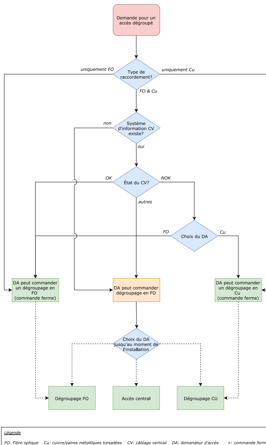
Graphique 4-9 : Obligation d'accès en fonction de l'infrastructure existante
