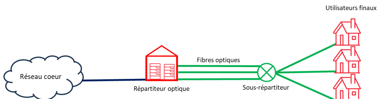
Graphique 2-7 : La configuration du réseau FTTH-P2P
