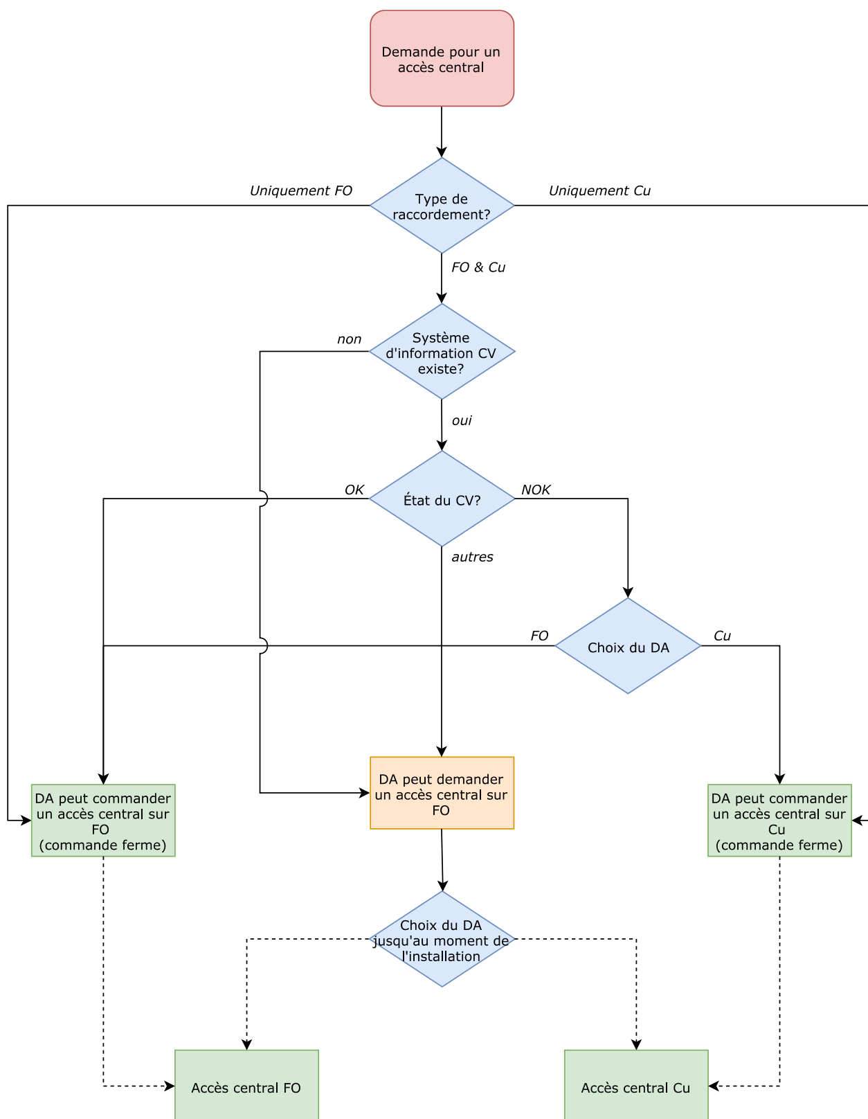
Graphique 5-6 : Obligation d'accès en fonction de l'infrastructure existante
