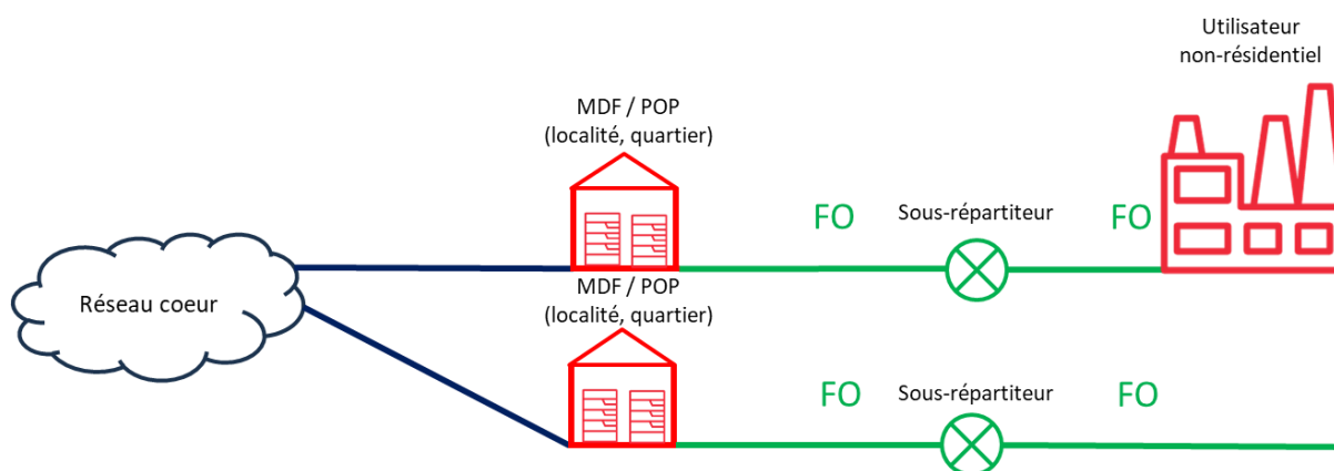
Graphique 2-9 : La configuration du réseau FTTO
